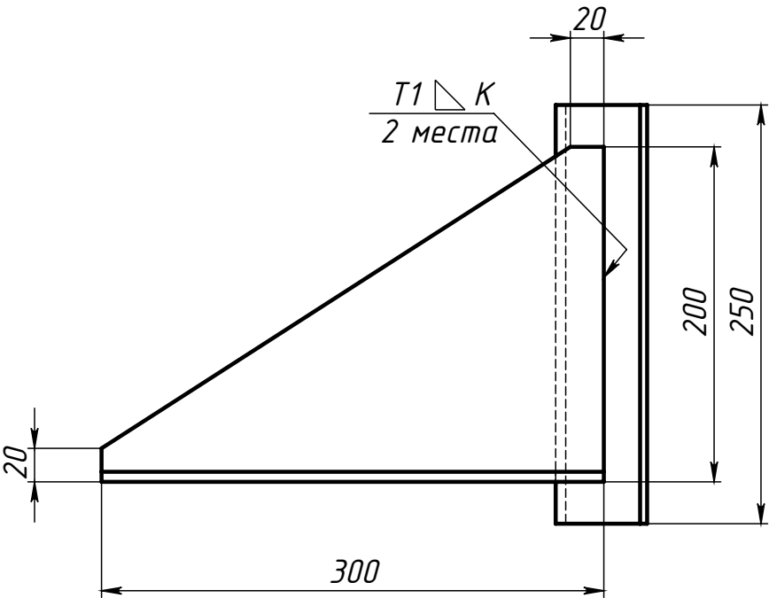
Поз.1 (Основание)
