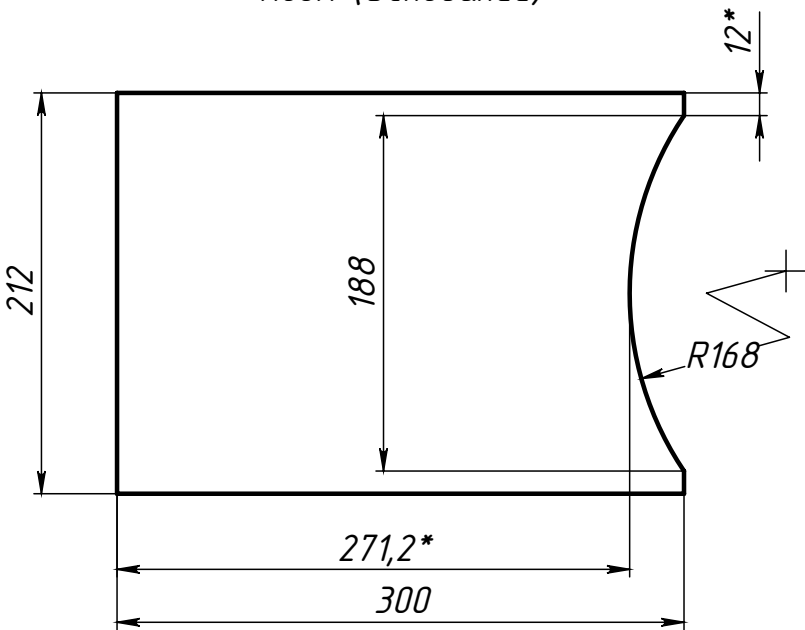
Поз.1 (Основание)
