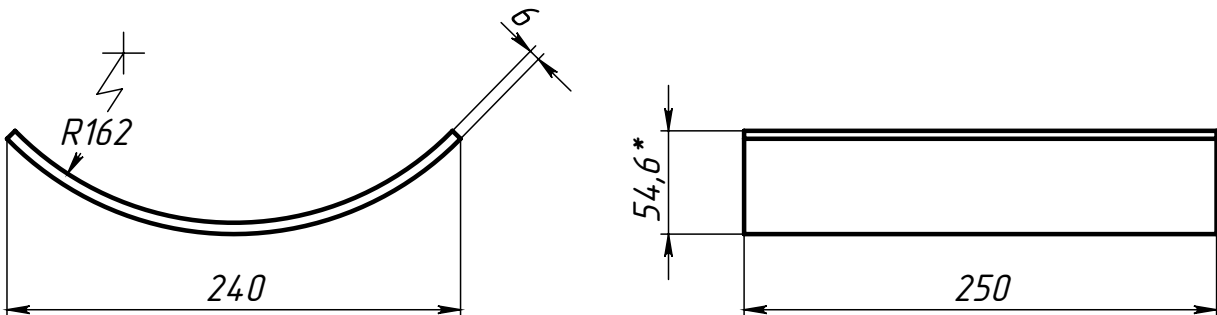
Поз.3 (Ложемент)
